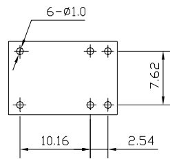
安装图
